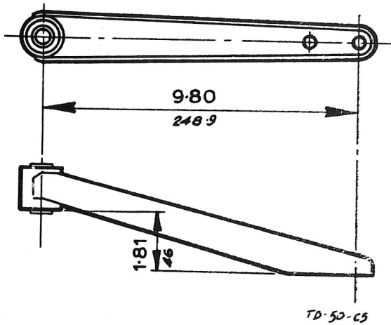
Fig. 5. UPPER WISHBONES
