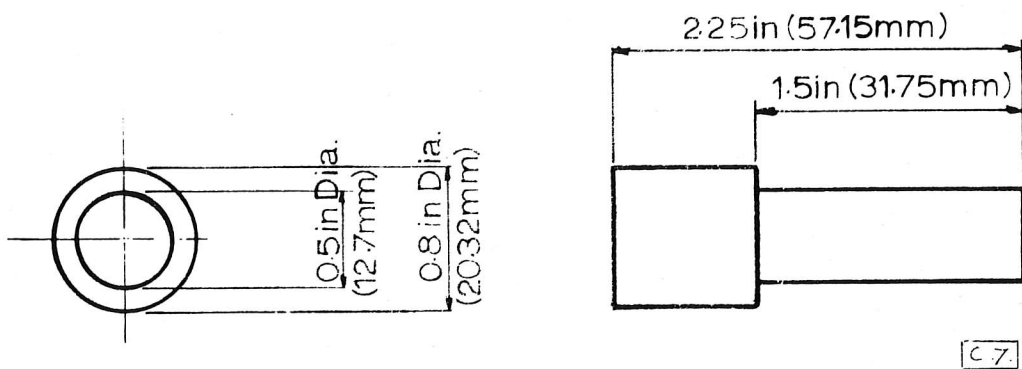
Fig. 9 MANDREL
